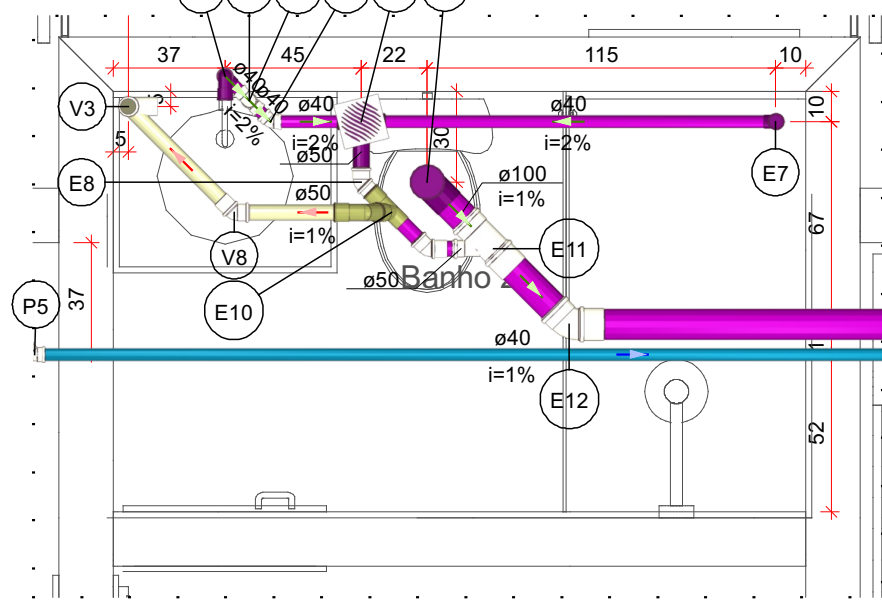
Detalhe Sanitário-4 Escala 1:25
