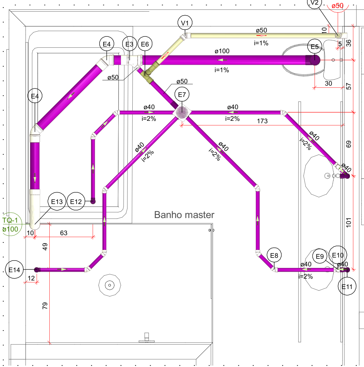
Detalhe Sanitário-6 Escala 1:25
