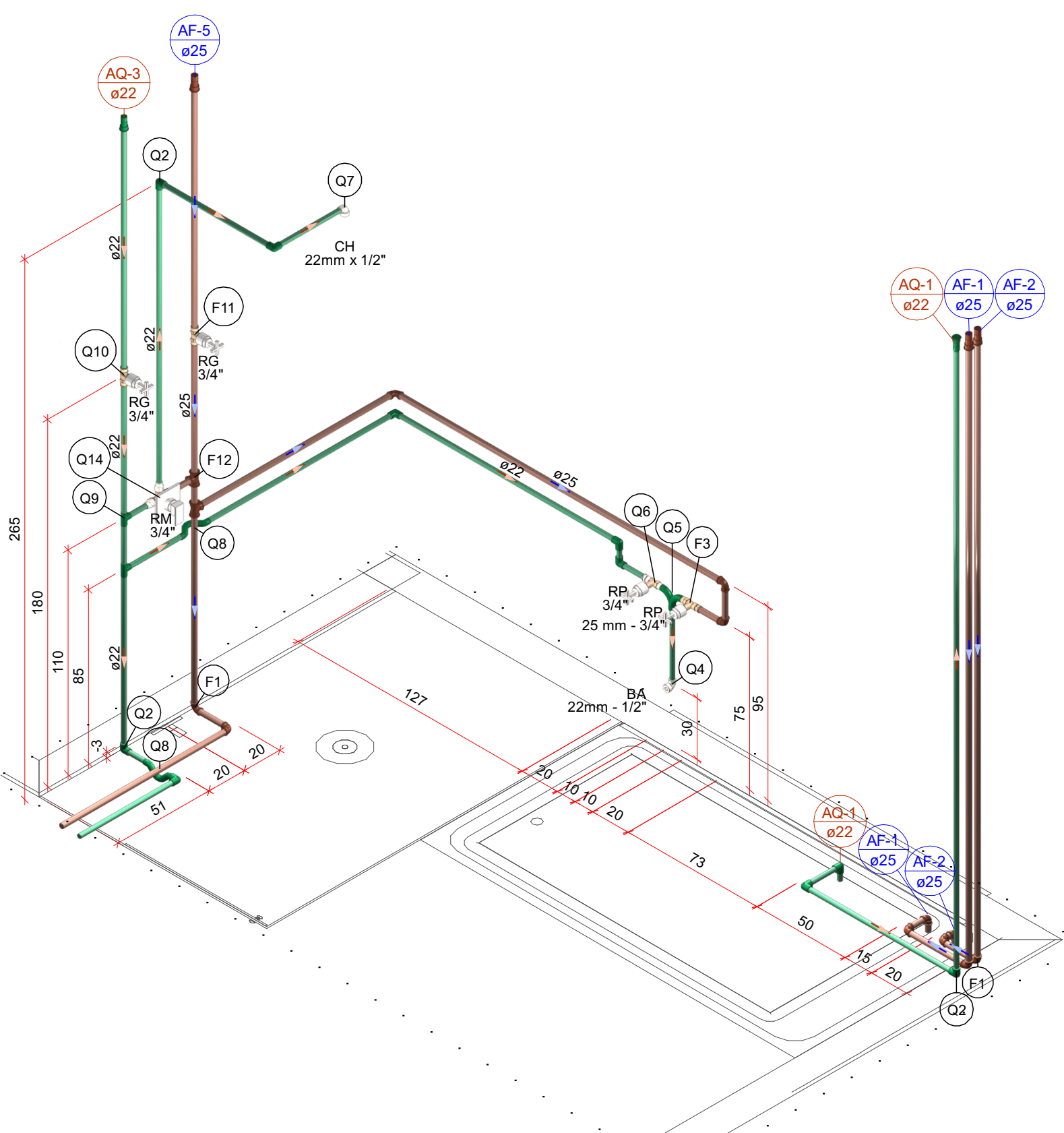
Detalhe Hidráulico-9 Escala 1:25
