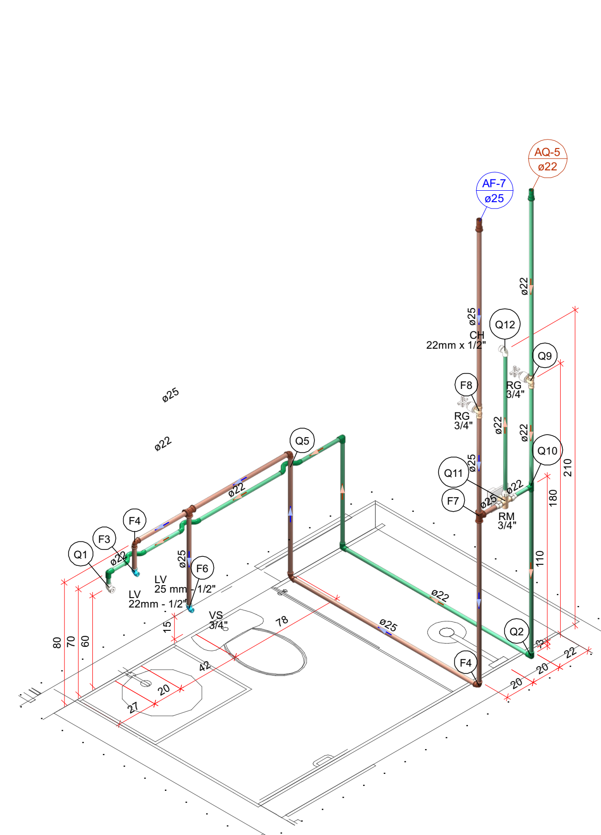
Detalhe Hidráulico-10 Escala 1:25
