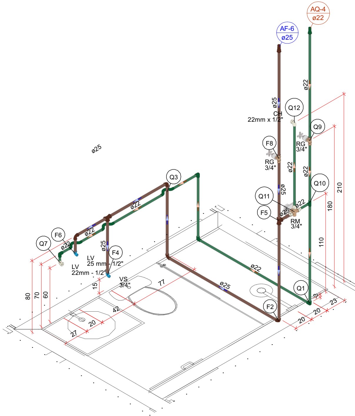
Detalhe Hidráulico-8 Escala 1:25
