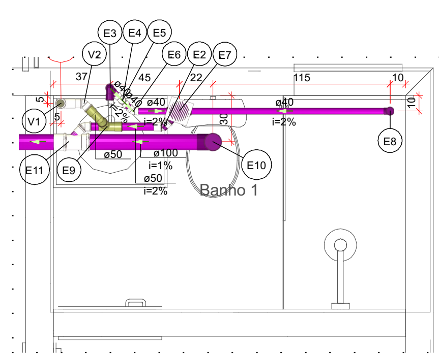
Detalhe Sanitário-7 Escala 1:25
