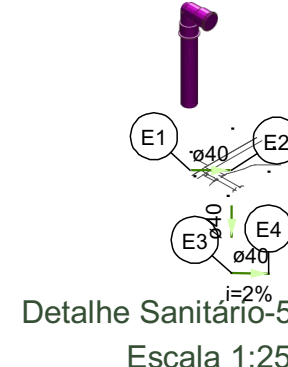
Detalhe Sanitário-5 Escala 1:25
